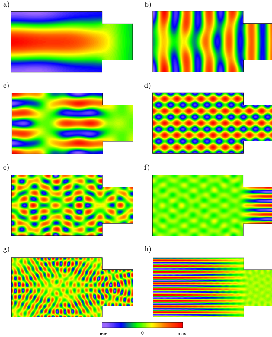
FIG. 3. Contour maps of eigenfunctions \Psi_\kappa for the modal number \kappa : a) 9, b) 50, c) 60, d) 154, e) 200, f) 271, g) 500, h) 652. Frequencies f_\kappa for these functions are (in Hz): a) 34.5, b) 93.4, c) 104, d) 171.5, e) 195.1, f) 229.2, g) 313.9, h) 360.2.
